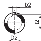
Albero uscita cavo Hollow output shaft Abtriebshohlwelle
