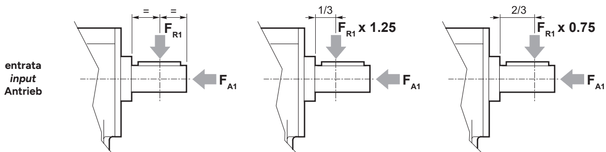
Carichi radiali F_{R1} e assiali F_{A1} sull'albero entrata [N]
